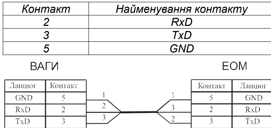
Рис. 1. Схема паяння кабелю для з'єднання ваг з IBM PC.
